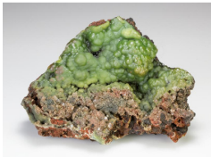
Arsendescloizite - Mexico
